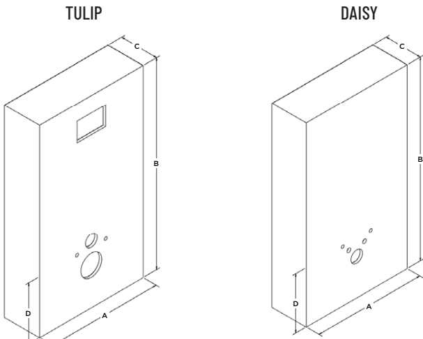
Tolérances dimensionnelles +/- 5 mm.
