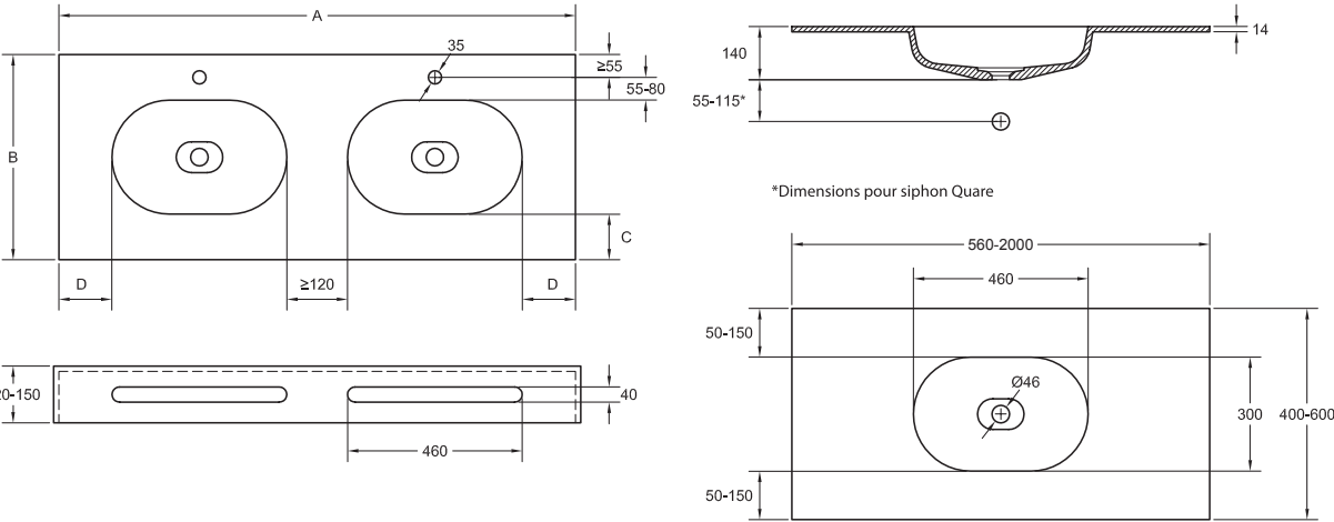
Elements de fixation inclus (Autoportant)
