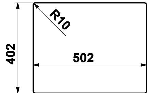
Foro Sottotop
