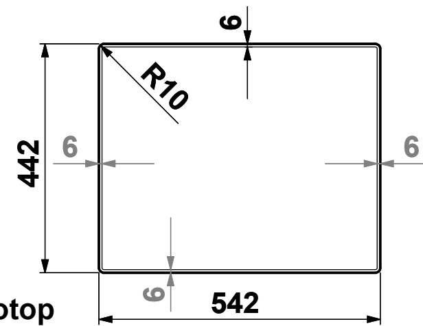
Foro Sottotop
